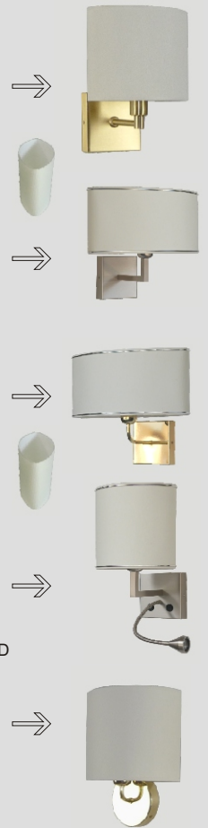
Wandleuchte, Nickel-matt-gebürstet 1xE27, 1xLED-Flexarm, 1 Watt, warm-weiß Höhe ca. 30 cm, Breite 21 cm, Tiefe 18 cm Schirm-oval, Chintz-champ. 21x14x17 cm 52308MM-503, Messing-matt 52308MP-503, Messing-polier 52308NM-503, Nickel-matt 52308CH-503, Chrom
